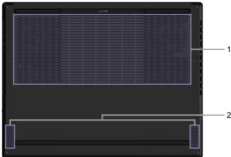
Рис. 6. Legion 9 16IRX8—вид снизу
